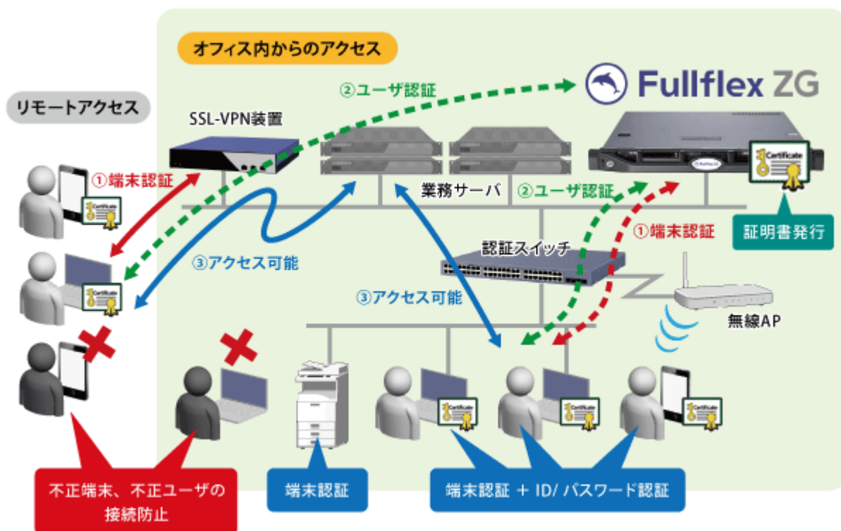
【不正防止アクセス防止認証統合ソリューション概念図】
