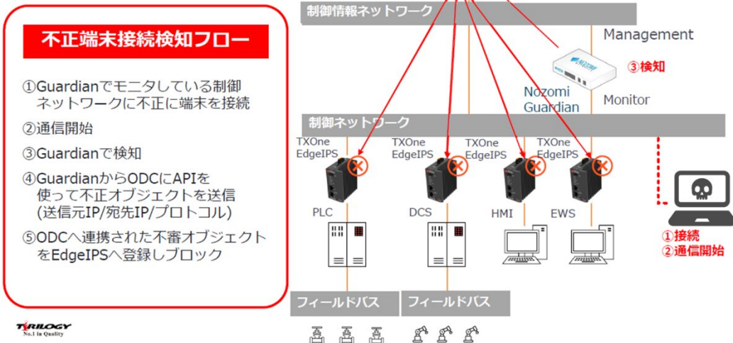
TXOne Networks Edge シリーズと Nozomi Networks Guardian の連携イメージ
